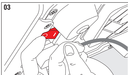
Fig. 03: Apagar el dispositivo ionizante girando el interruptor On/Off a la posición 0 .
